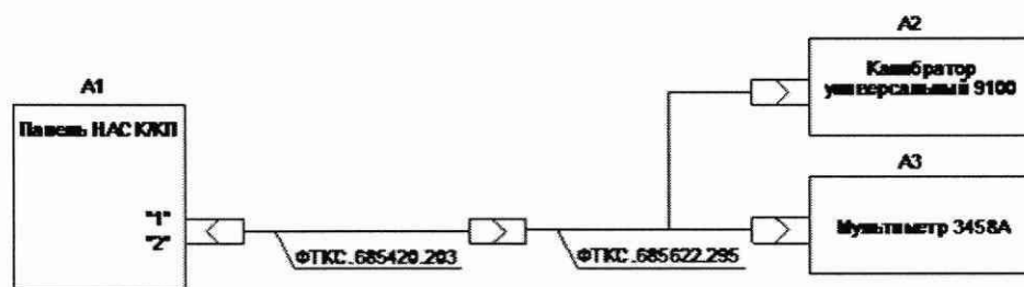
Рисунок 22 – Определение относительной погрешности измерений напряжения постоянного тока
