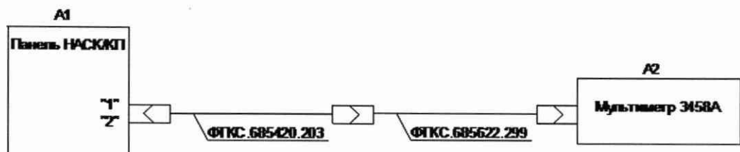
Рисунок 27 – Определение относительной погрешности воспроизведения и измерений напряжения постоянного тока источников питания
