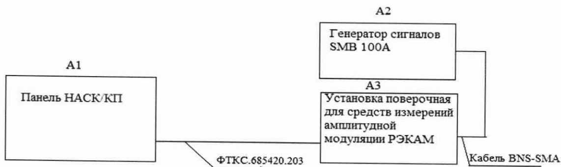
Рисунок 4 - Определение абсолютной погрешности установки коэффициента АМ в режиме внутренней синусоидальной амплитудной модуляции
