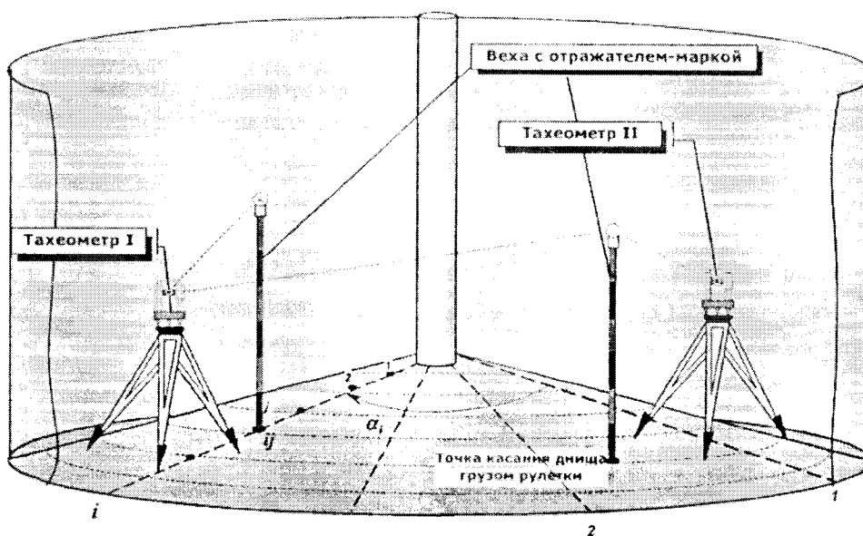
Рисунок А.6 Определение параметров дна резервуара при наличии в резервуаре центральной трубы
