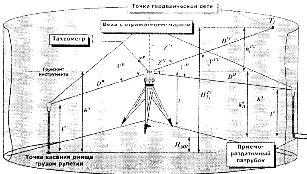
Рисунок А.3 Определение абсолютной высоты точки геодезической сети и „мертвой” полости относительно точки касания дна груза рулетки при установке тахеометра внутри резервуара
