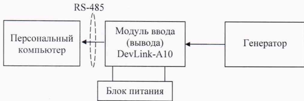
Рисунок А.4.2 – Схема соединений при проверке счёта импульсов (при наличии только модулей ввода (вывода) DevLink-A10)
