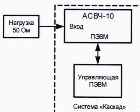
Рисунок 6 – Схема стенда поверки
