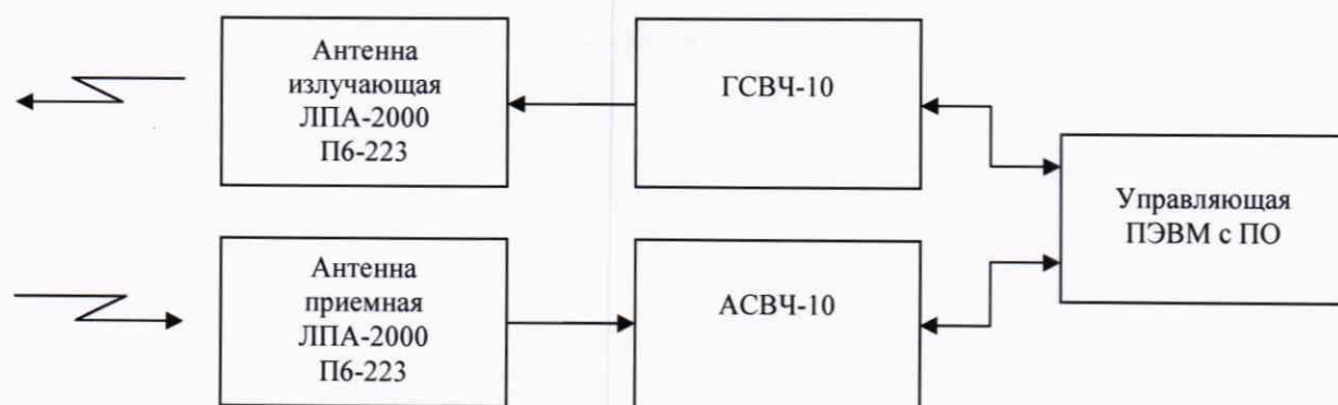
Рисунок 1 – Схема измерений
