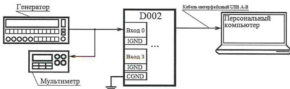
Рисунок 2 – Схема измерений
