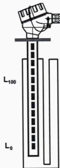
Рис. 3 - Проверка уровнемеров на установках с непосредственным изменением уровня в виде сообщающихся сосудов
