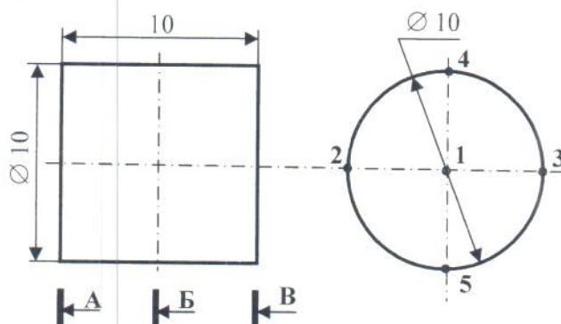
Рисунок А1 – Схема расположения точек контроля постоянной соленоида в его рабочей зоне.
