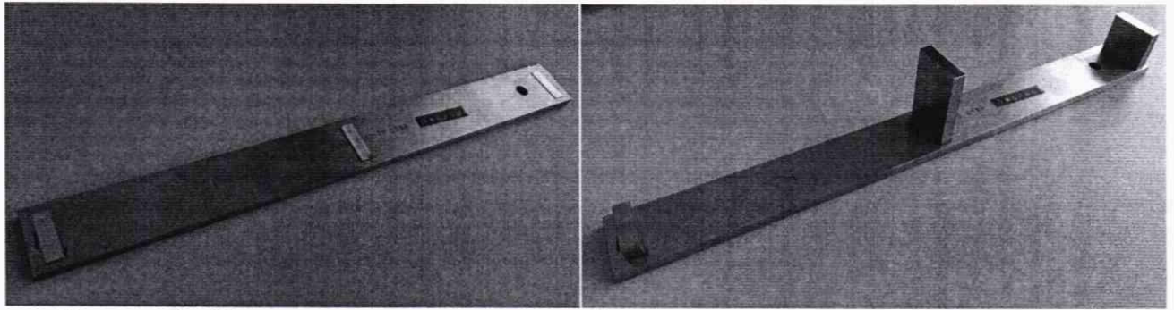
Рисунок 3 – Установка концевых мер на рабочую поверхность линейки поверочной
