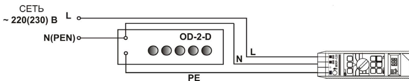
Рисунок 5 – Структурная схема определения абсолютной погрешности измерения напряжения прикосновения.
