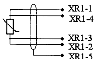
Рисунок 1 – Схема подключения датчиков датчиков с выходом по сопротивлению для измерений по схеме «одиночный тензорезистор»
