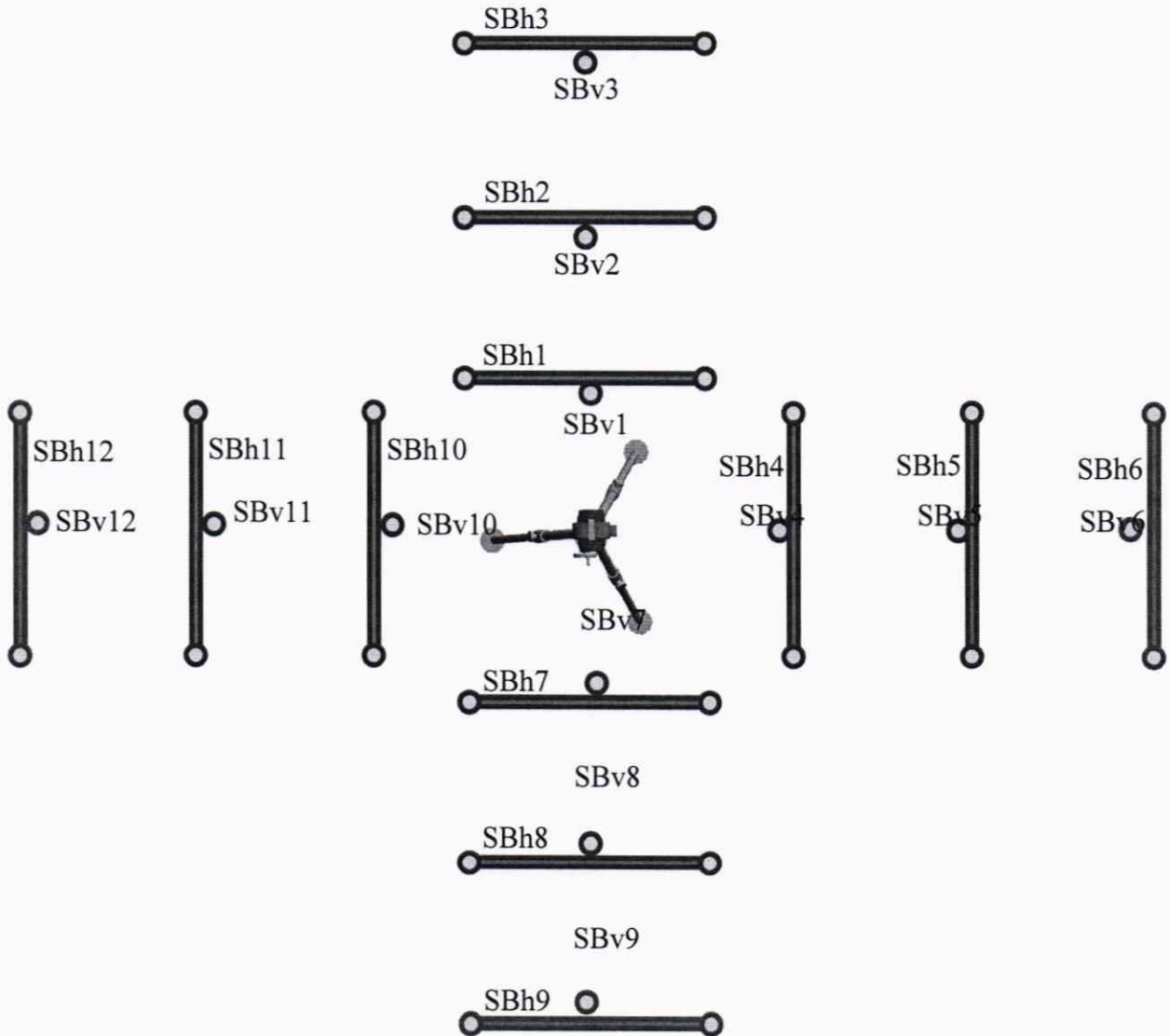
Рисунок 1 – Схема установки меры относительно системы. Вид сверху
