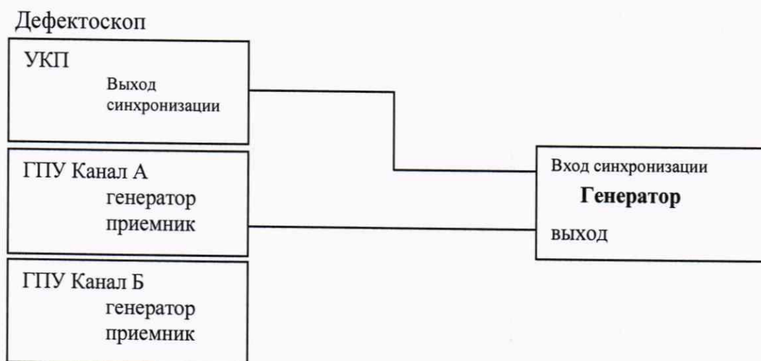
Рисунок 3 – Схема соединения для определения абсолютной погрешности измерений длительности временных интервалов
