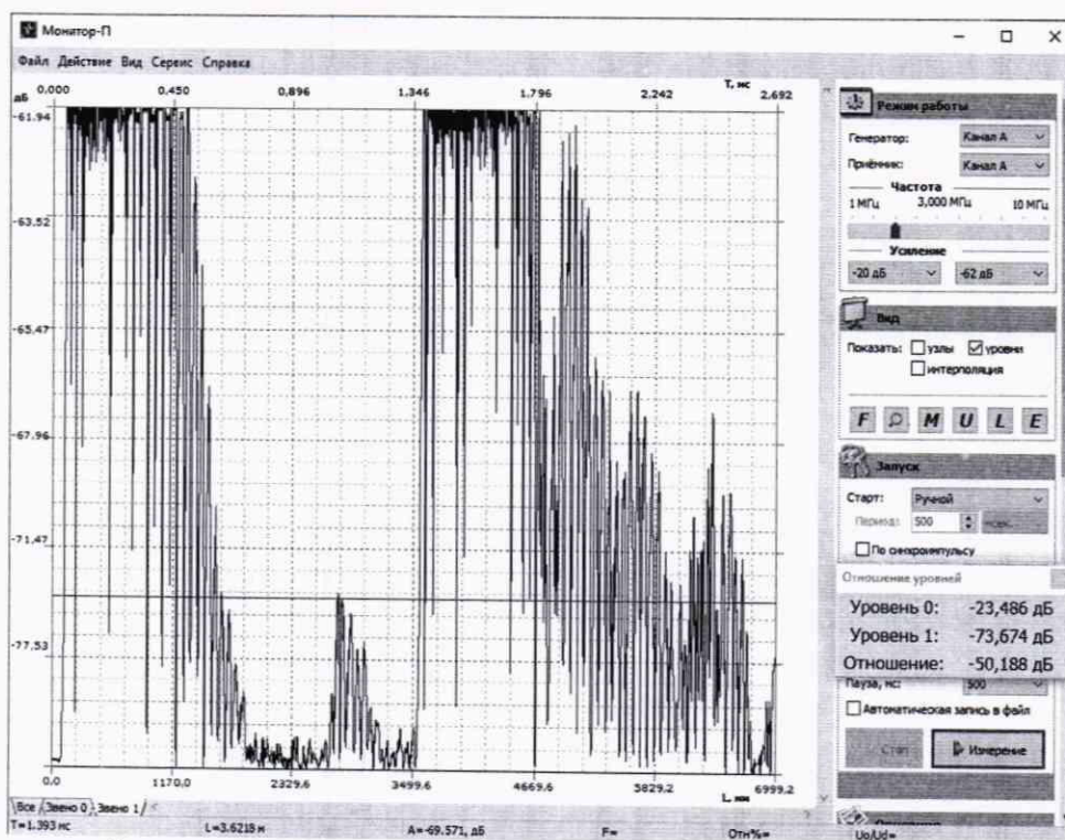
Рисунок 2 – Регистрация сигнала от дефекта на развертке
