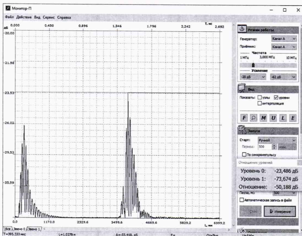
Рисунок 1 – Регистрация донного сигнала на развертке
