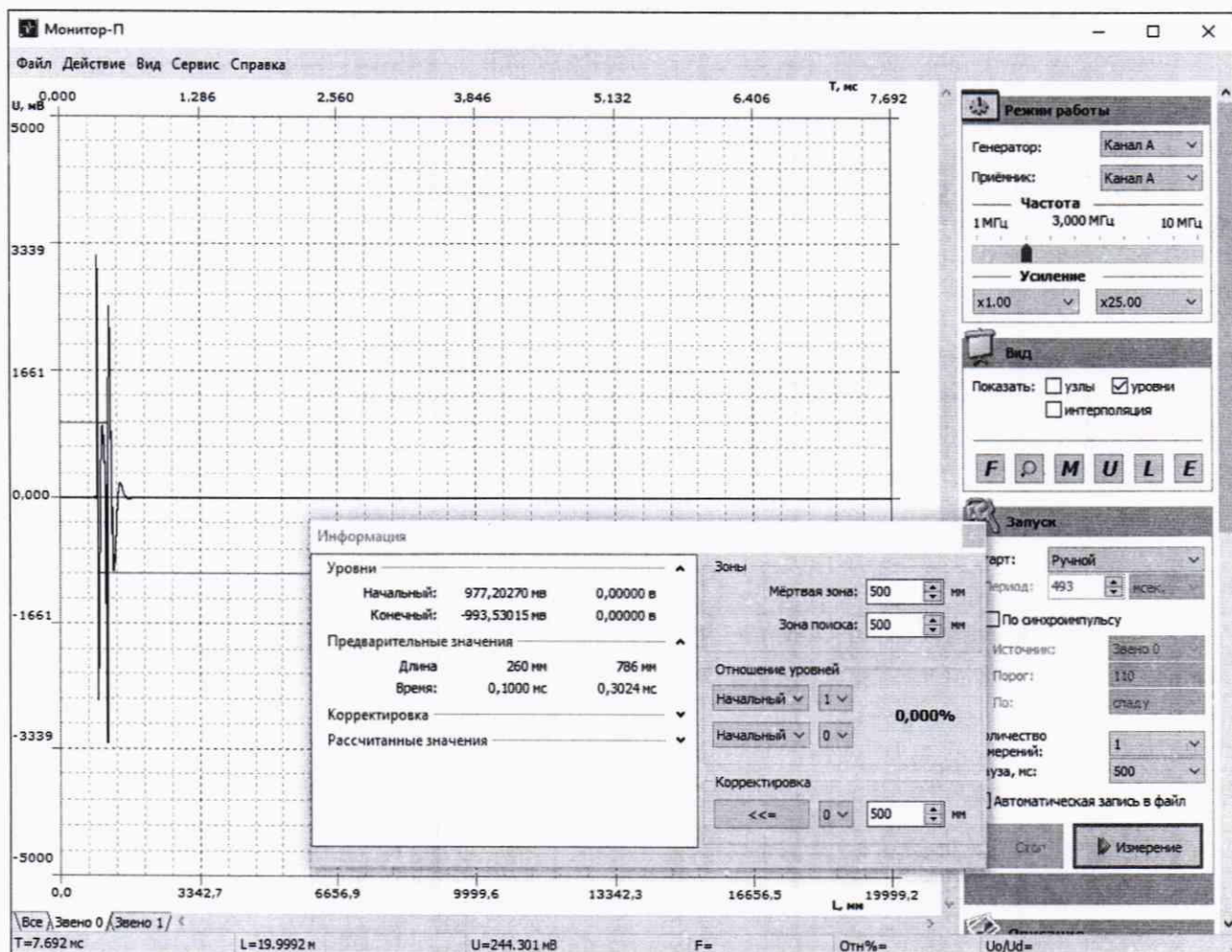
Рисунок 4 – Установка уровня
