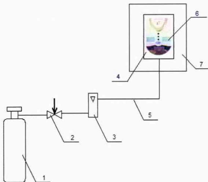
Рис. 1 - Схема подачи ПГС к сигнализатору
