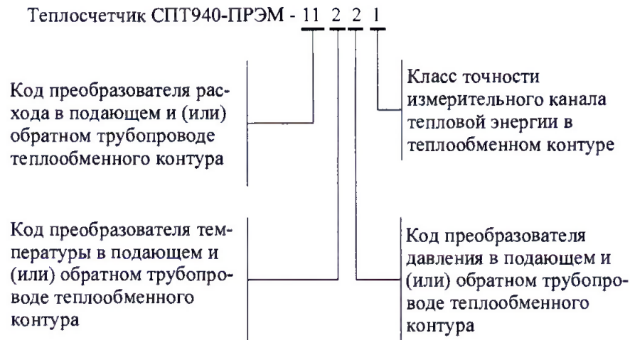
Рисунок 2.1 – Структура обозначения теплосчетчиков
