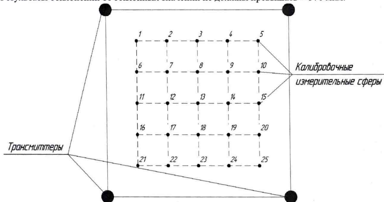
Рисунок 1- Схема определения допустимой абсолютной погрешности объемных (3D) измерений ( 2\sigma )
