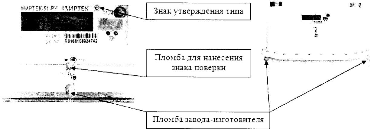
Рисунок Б.1 – Общий вид счетчиков и схема нанесения знака поверки
