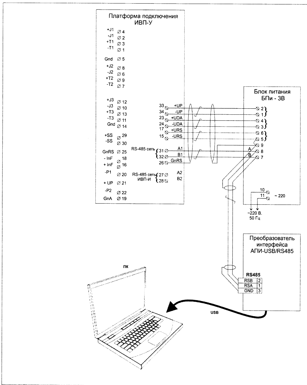
Рисунок Г.2 — Схема подключения АТ-Т к ПК в случае реализации аппаратно программной версии АПВ-1
