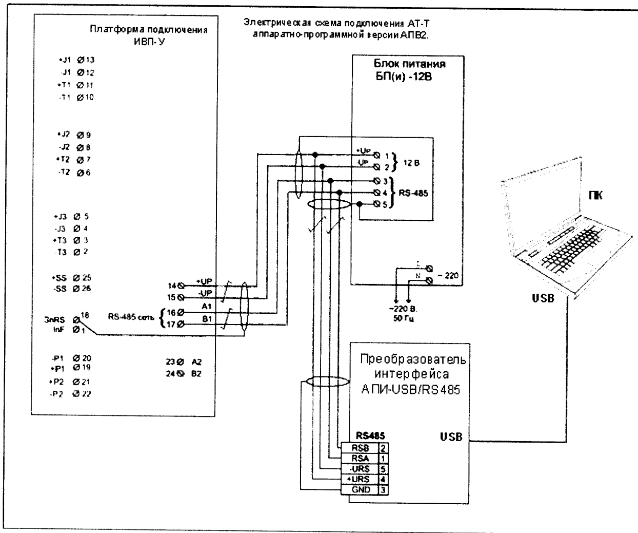
Рисунок Д.2 — Схема подключения АТ-Т к ПК в случае реализации аппаратно-программной версии АПВ-2
