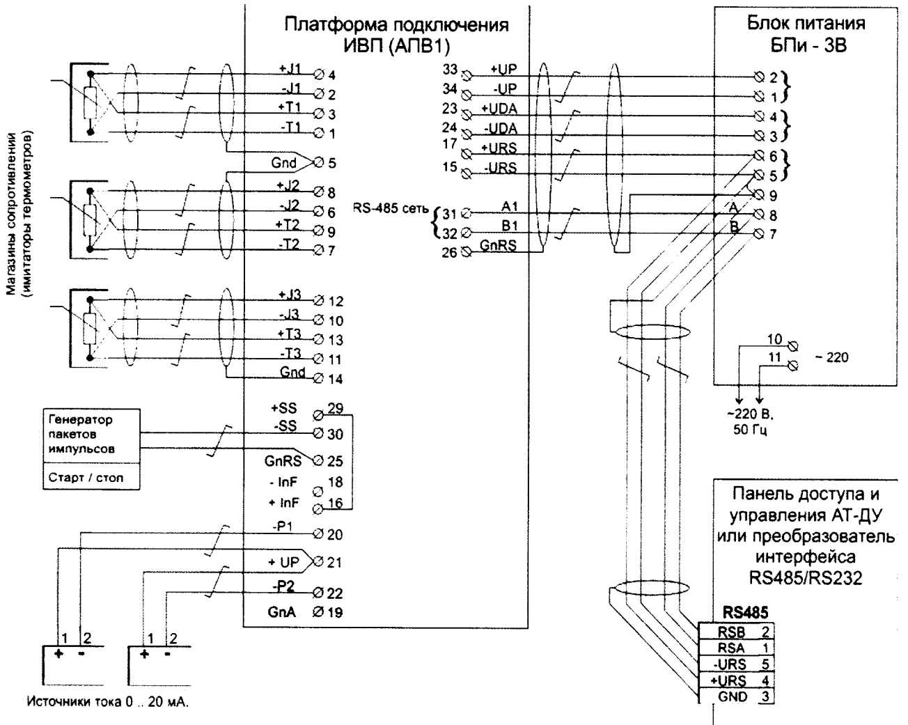
Рисунок А.1 - Схема подключения средств поверки каналов температуры и давления (без датчиков температуры и давления) к ИВП АПВ1
