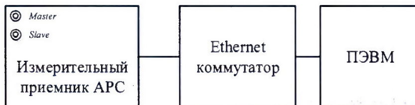
Рисунок 2. Схема подключения для определения среднего уровня собственных шумов
