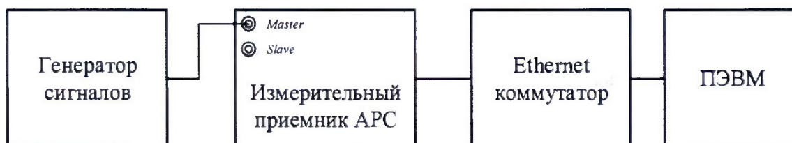
Рисунок 3. Схема подключения для проверки уровня избирательности, уровня спектральной плотности мощности фазовых шумов, динамического диапазона
