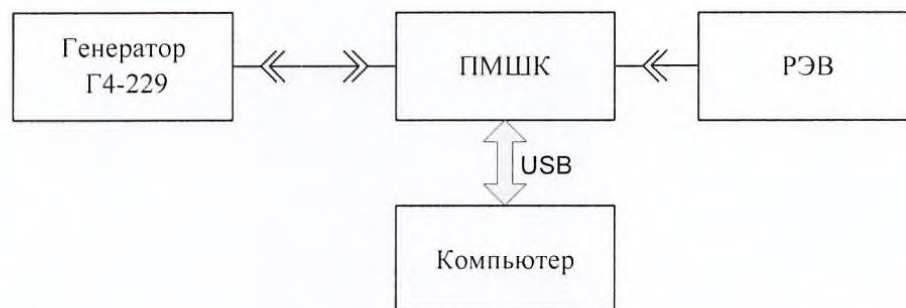
Рисунок 6 - Схема для определения модуля эффективного коэффициента отражения выхода преобразователя ПМШК
