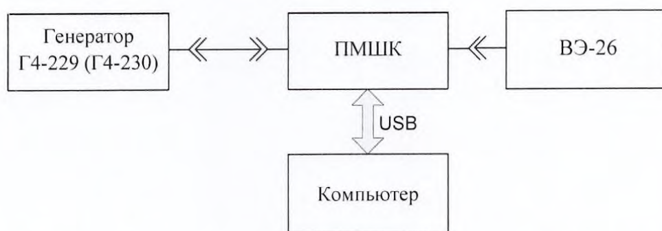
Рисунок 9 – Схема определения калибровочного коэффициента преобразователя ПМШК
