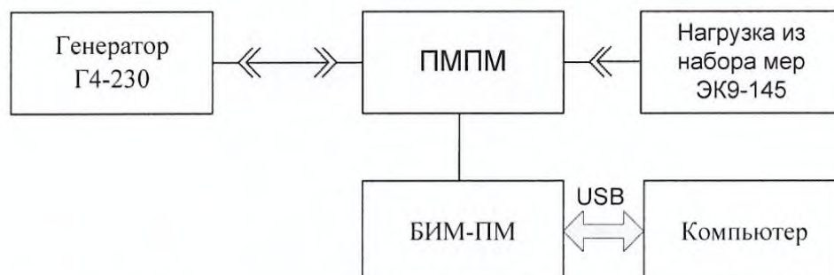
Рисунок 11 – Схема определения относительной погрешности измерения КСВН для преобразователей ПМППМ-1 и ПМППМ-2
