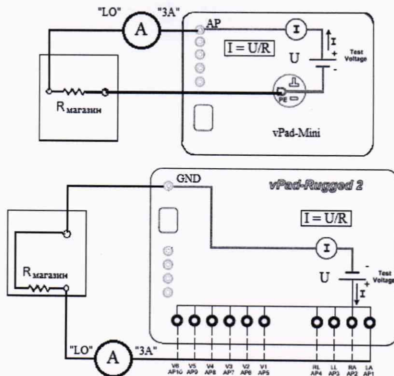
Рисунок 6 - Схема соединения при проверке режима Applied Part Leakage – MAP Test (Voltage).
