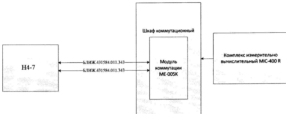
Рисунок 15 - Схема поверки электрической части ИК температуры
