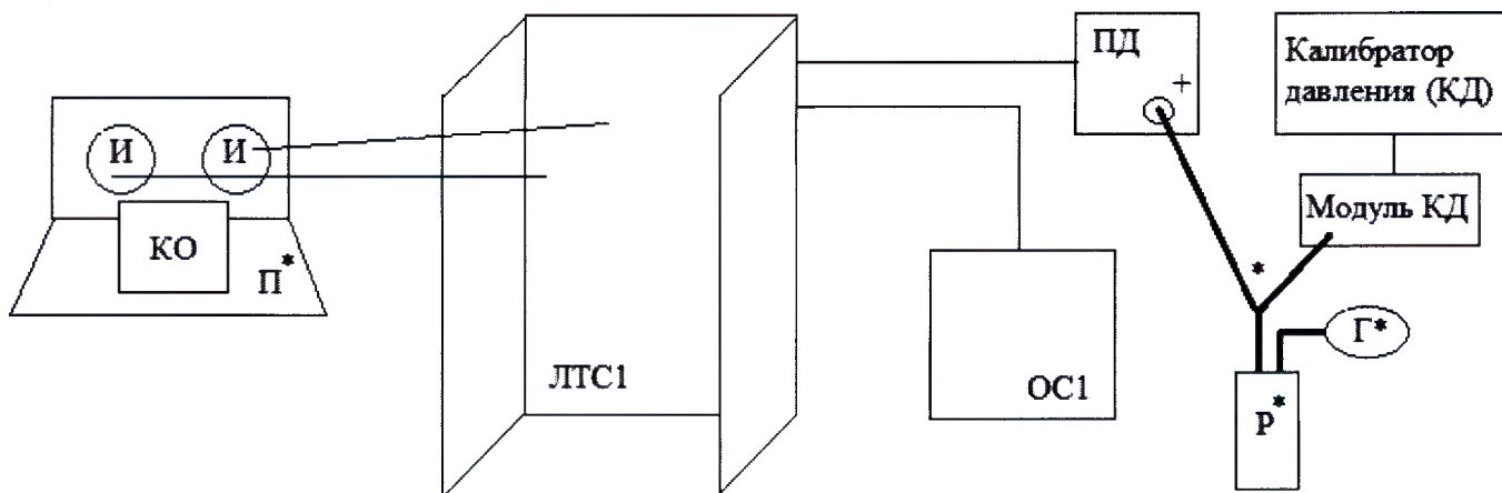
Рисунок 1 Схема подключения СИ при проверке
