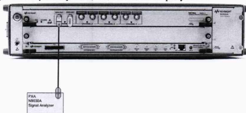
Рисунок 2. Измерение интермодуляционных искажений.
