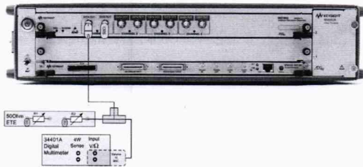
Рисунок 1. Измерение погрешности установки выходного напряжения.
