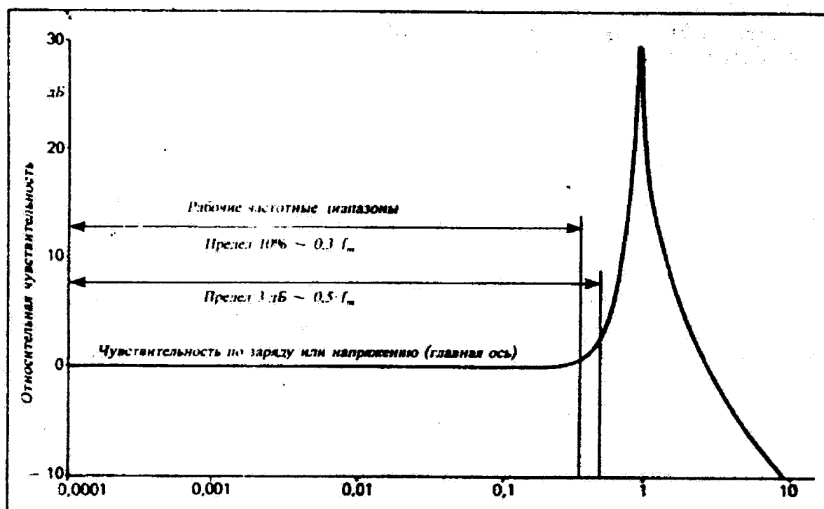
Кривая амплитудно-частотной характеристики (АЧХ) датчика
