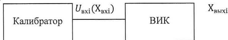
Рисунок 2 - Схема подключения при определении МХ ВИК преобразования сигналов напряжения переменного тока
