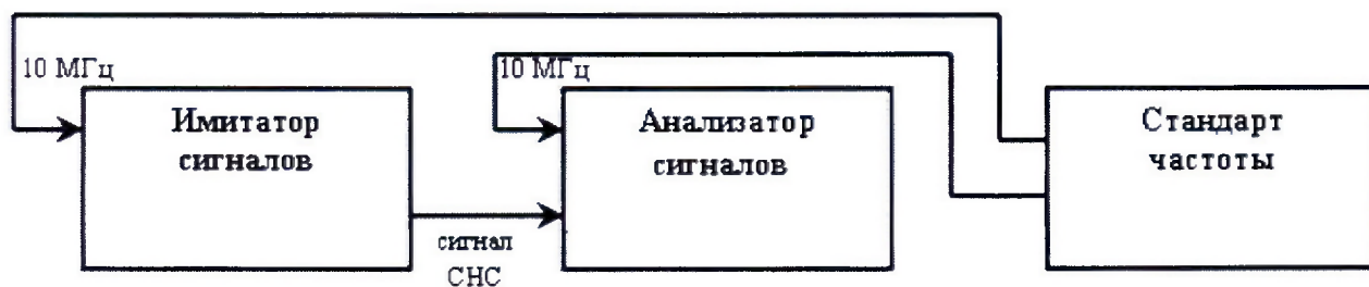
Рисунок 1 – Схема измерений
