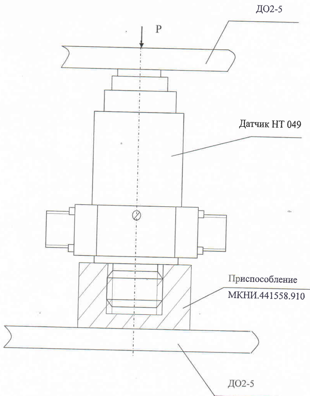
Рисунок 2 – Схема установки датчика на динамометр образцовый ДО 2-5
