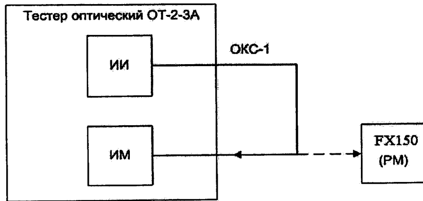
ИИ – источники излучения оптического тестера ОТ-2-3А; ИМ – измеритель оптической мощности оптического тестера ОТ-2-3А; ОКС-1 – оптический кабель соединительный; PM – измеритель оптической мощности прибора FX150
