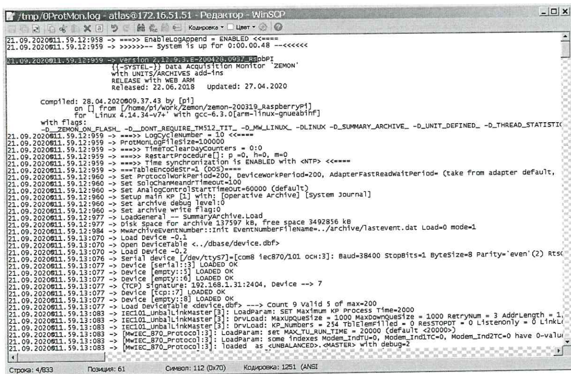
Рисунок 5 – Лог-файл OProtMon.log
