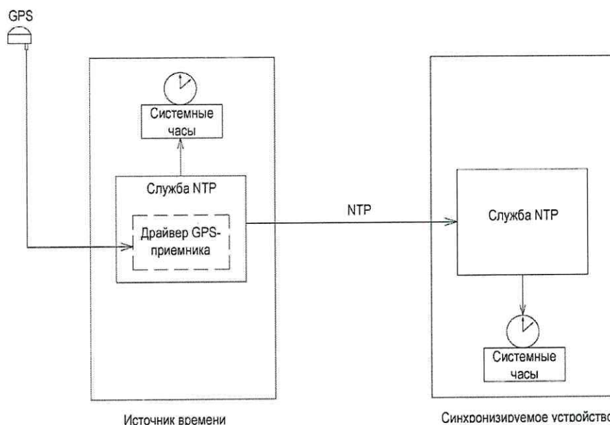
Рисунок 10 – Схема для проверки пределов допускаемой абсолютной среднесуточной погрешности хода часов УСПД без внешней синхронизации
