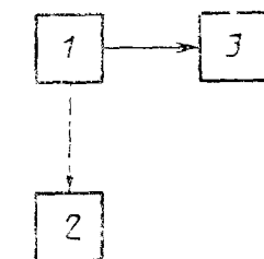
1—образцовая установка К2-38; 2—электронно-счетный частотомер; 3—поверяемый АС
