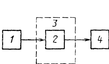
1—генератор ВЧ или СВЧ сигнала; 2—входной аттенюатор АС; 3—поверяемый АС, 4—установка для поверки аттенюаторов
