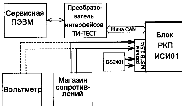
Рисунок 1 – Схема проверки блоков ИСИ01
