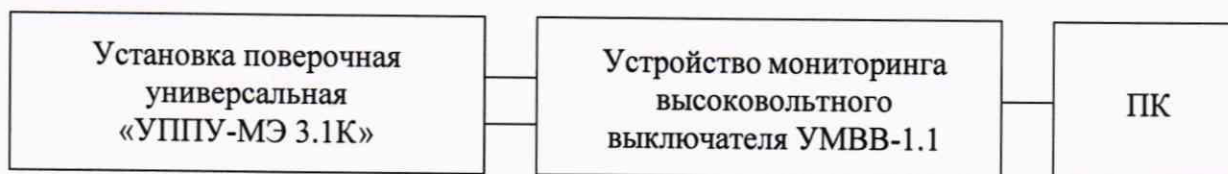
Рисунок 2 – Схема подключения для определения относительной погрешности измерений силы переменного тока частотой 50 Гц
