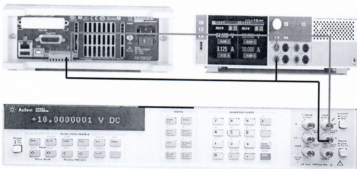
Рисунок 8 – Структурная схема соединения СИ для определения абсолютной погрешности измерений постоянного напряжения
