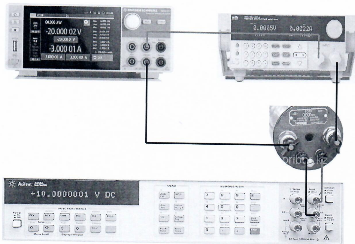
Рисунок 5 – Структурная схема соединения СИ для определения нестабильности силы постоянного тока на выходе при изменении напряжения на нагрузке от 10 % до 90 %
