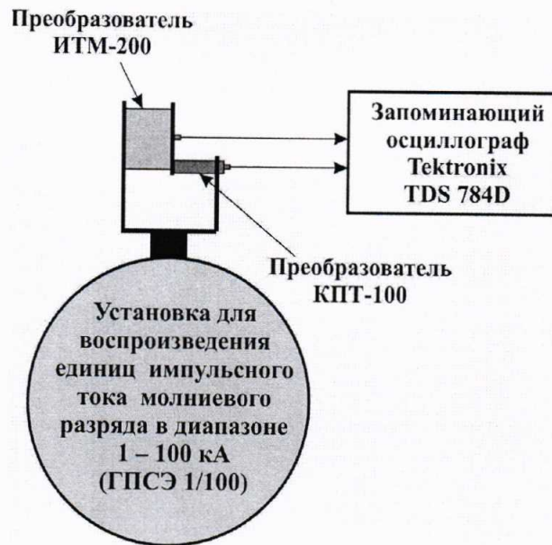
Рисунок 1 – Схема исследований при определении характеристик преобразователей с использованием установки ГПСЭ 1/100 для воспроизведения единицы импульсного тока в диапазоне от 1 до 100 кА
