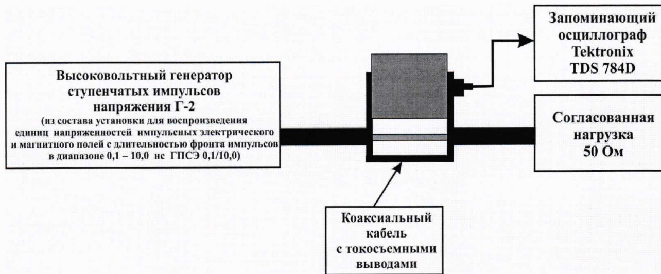
Рисунок 3 – Схема измерений при определении времени нарастания переходной характеристики преобразователя ИТМ-200
