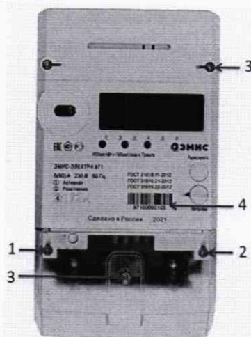
Рис. 1 – Схема пломбировки счётчиков ЭМИС-ЭЛЕКТРА 971 исполнения «X»
