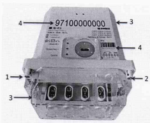
Рис. 2 – Схема пломбировки счётчиков ЭМИС-ЭЛЕКТРА 971 исполнения «С»
