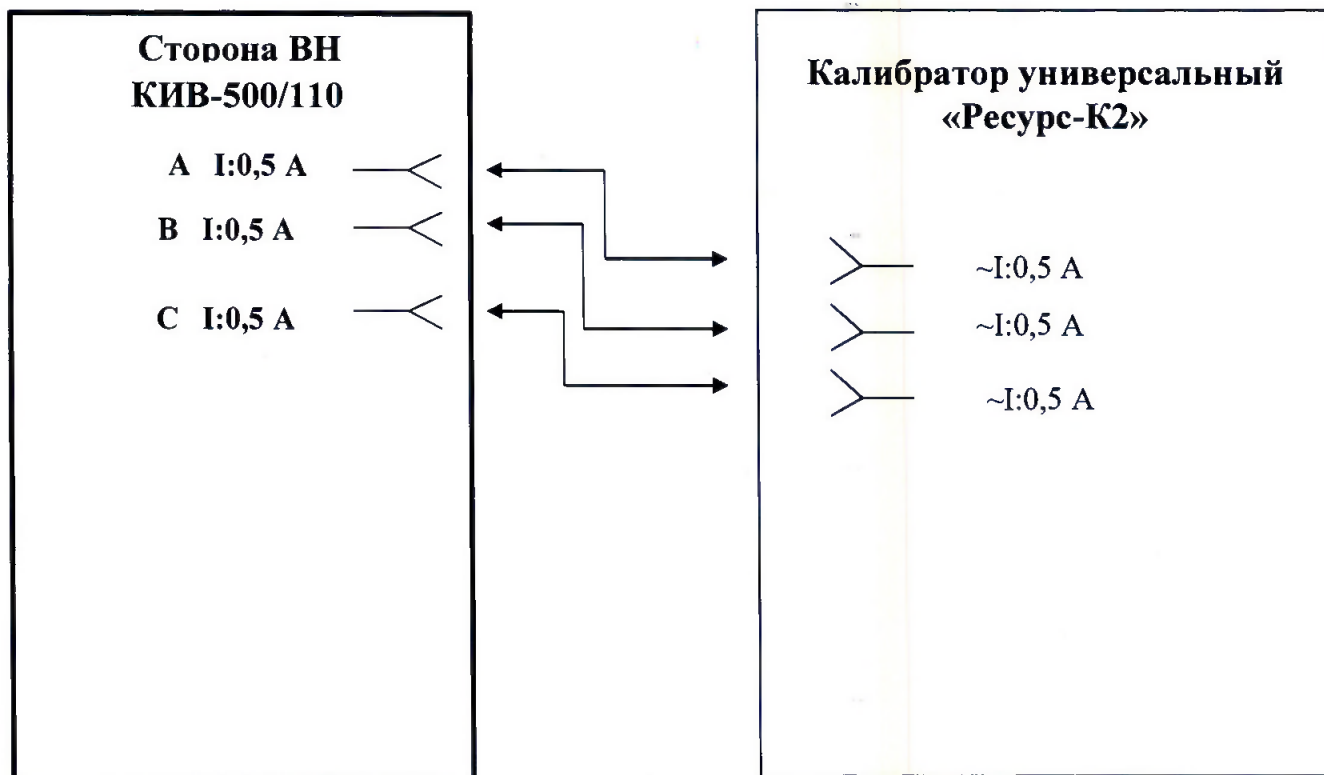
Рисунок А1 - Схема подключения прибора измерительного КИВ-500/110 (по стороне ВН) к калибратору универсальному «Ресурс-К2» для определения допустимой относительной погрешности измерений силы переменного тока (тока утечки)
