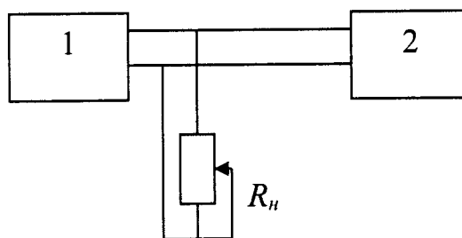
1 — поверяемый источник 2 — осциллограф Fluke 124 R_n — нагрузочный реостат
