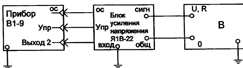
Рисунок 8 - Схема электрическая структурная подключения приборов для определения основной погрешности измерения напряжения переменного тока синусоидальной формы до 100V
