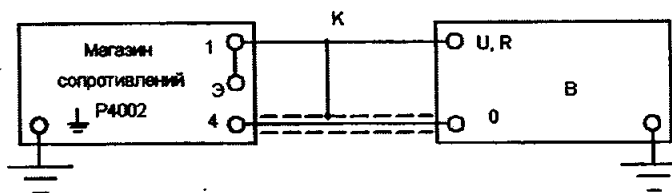
Рисунок 21 - Схема электрическая структурная подключения приборов для определения основной погрешности измерения электрического сопротивления на пределе 2000 кΩ в поверяемых точках 1500 и 1900 кΩ
