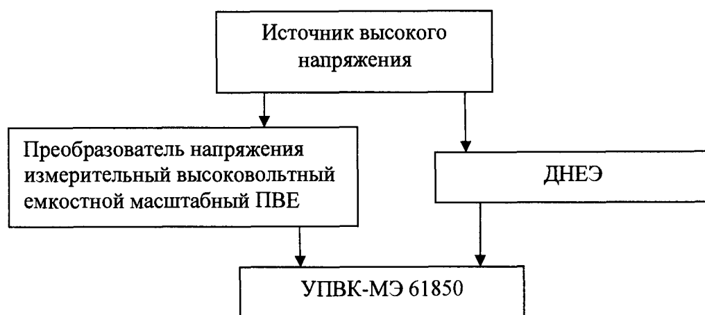
Рисунок 2. Схема для определения погрешности коэффициента масштабного преобразования и угла фазового сдвига синусоидального напряжения
