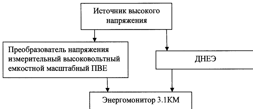
Рисунок 1. Схема для определения погрешности коэффициента масштабного преобразования напряжения
