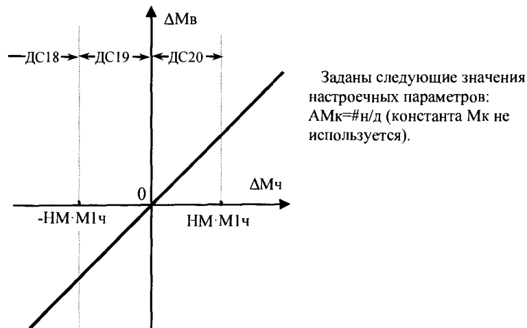
Рисунок 7.5 – Контроль разности часовых масс \Delta M_{ч} = (M_{1ч} - M_{2ч})
