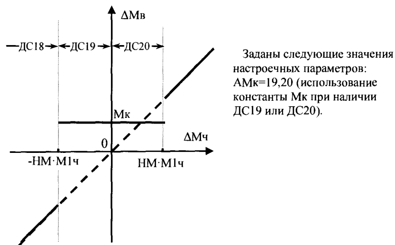
Рисунок 7.6 – Пример использования алгоритмов подстановок по результатам контроля разности часовых масс
