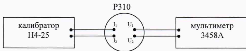
Рисунок 8 - Схема соединений при определении относительной погрешности воспроизведения силы постоянного электрического тока
