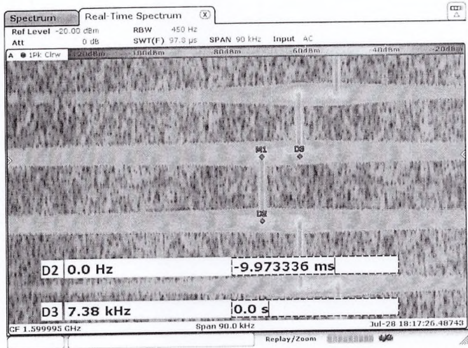
Рисунок 6 – Пример записи цифрового потока принимаемого сигнала
