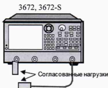
Рисунок 7 - Схема для определения уровня собственных шумов
