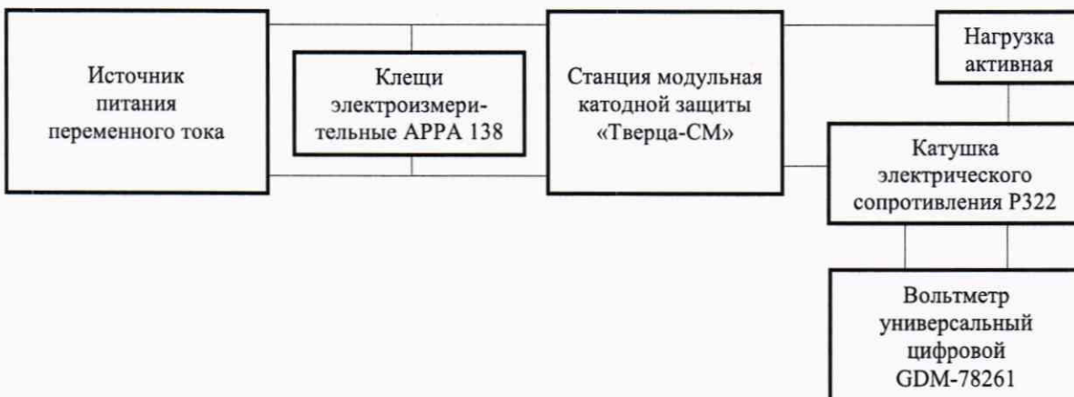
Рисунок 1 – Структурная схема
