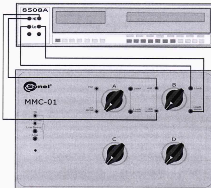
Рисунок 4 - Структурная схема определения среднего значения и вариации начального сопротивления, абсолютной погрешности воспроизведения электрического сопротивления мер ММС-01. (отдельные разъемы декады В).
