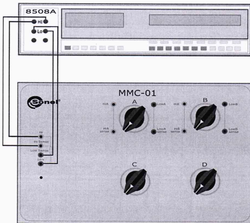
Рисунок 1 - Структурная схема определения среднего значения и вариации начального сопротивления, абсолютной погрешности воспроизведения электрического сопротивления мер ММС-01. (общие разъемы).
