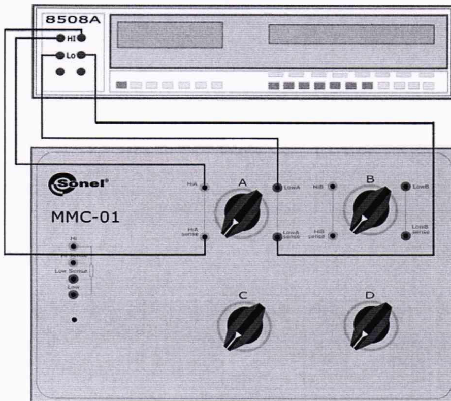
Рисунок 3 - Структурная схема определения среднего значения и вариации начального сопротивления, абсолютной погрешности воспроизведения электрического сопротивления мер MMC-01. (отдельные разъемы декады А).
