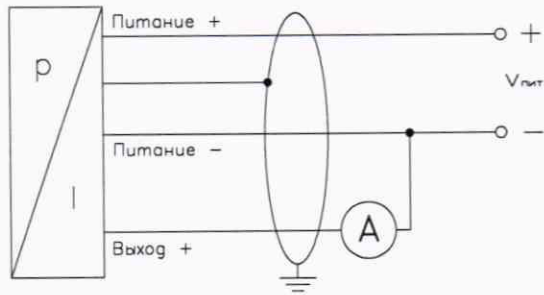
3-х пров. (вых. сигнал - ток)
