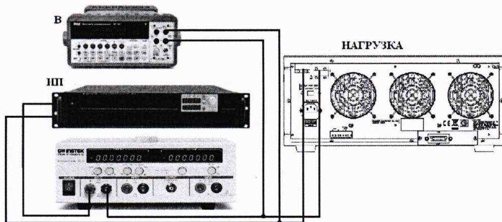
Рисунок 3 - Схема подключения приборов при определении абсолютной погрешности установки и измерений электрической мощности при работе в режиме стабилизации мощности
