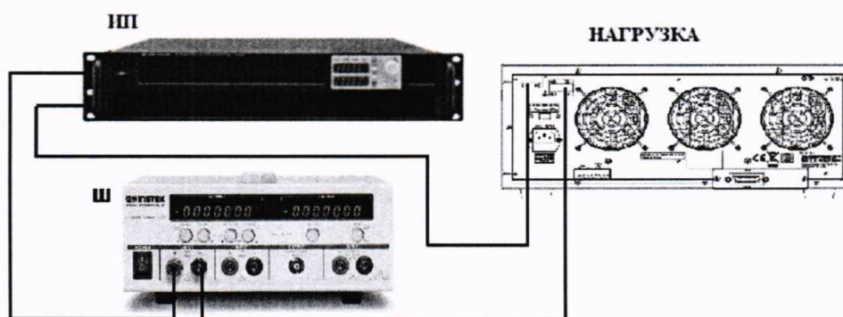
Рисунок 1 – Схема подключения приборов при определении абсолютной погрешности установки и измерений силы постоянного тока при работе в режиме стабилизации тока.
