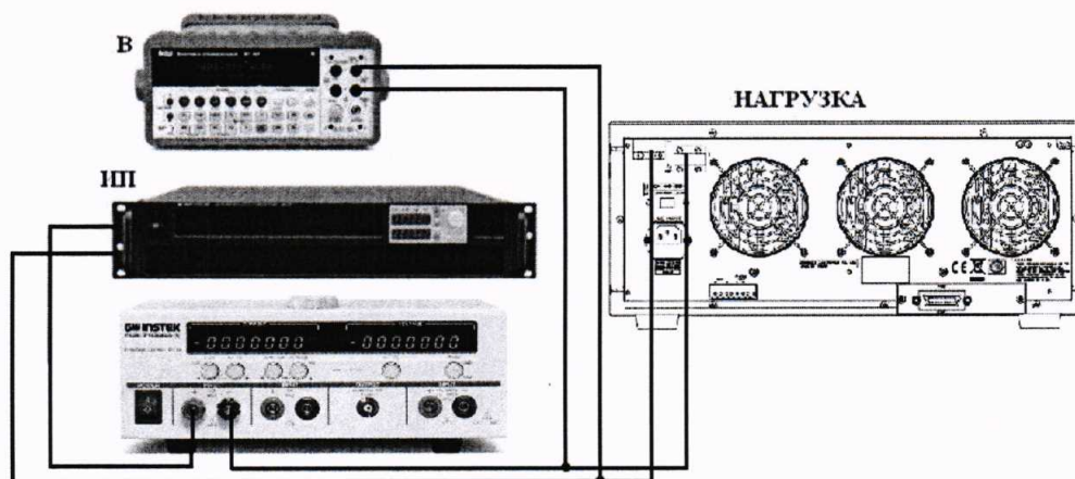
Рисунок 4 - Схема подключения приборов при определении абсолютной погрешности установки сопротивления при работе в режиме стабилизации сопротивления
