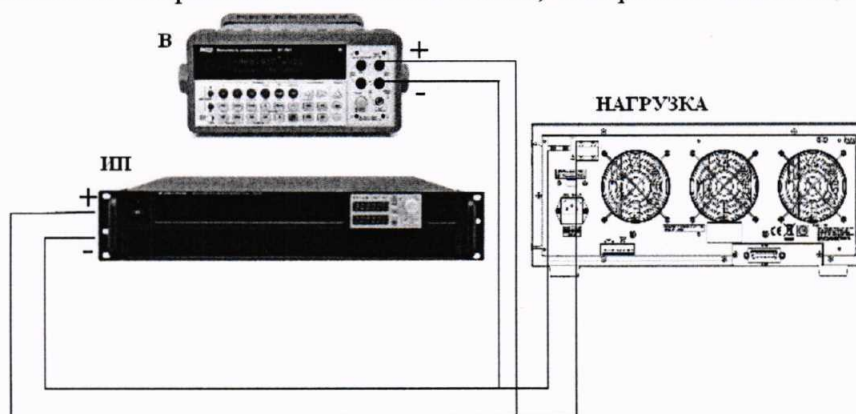
Рисунок 2 - Схема подключения приборов при определении абсолютной погрешности установки и измерений напряжения постоянного тока в режиме стабилизации напряжения.
