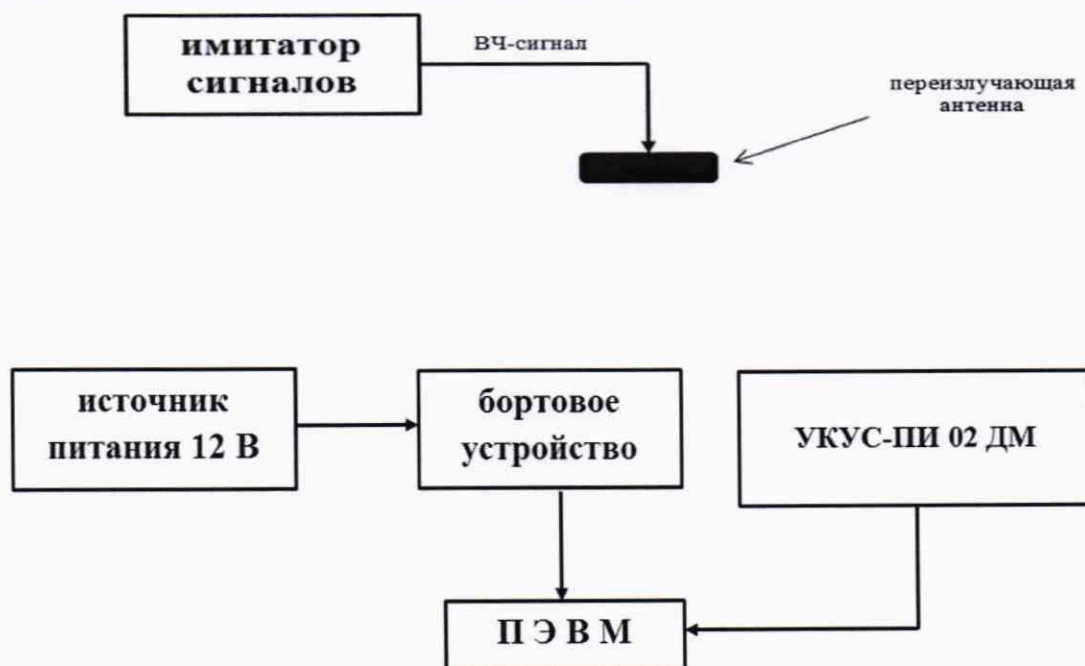
Рисунок 4 – Схема проведения измерений при периодической поверке устройств
