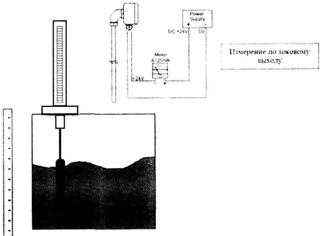
Рисунок 1 – Поверка уровнемера на поверочной установке с непосредственным изменением уровня жидкости
