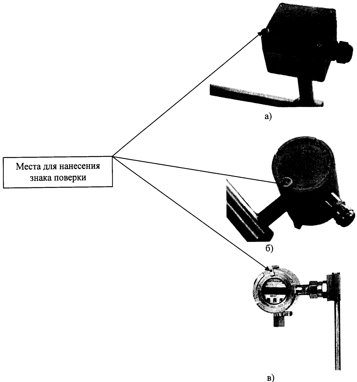
Рисунок Б.1 – Схема пломбировки от несанкционированного доступа, обозначение мест нанесения знака поверки
