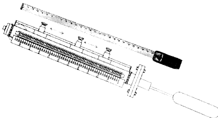
Рисунок 3 – Проверка уровнемера с помощью рулетки и магнитного замыкателя
