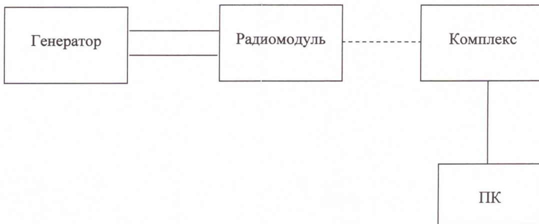
Рисунок 3 – Схема подключения для определения относительной погрешности измерения и преобразования количества импульсов электрического напряжения
